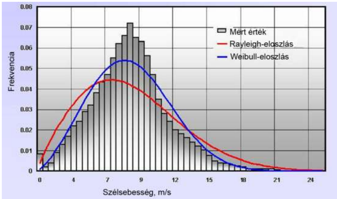
3.4. számú ábra: Szélsebesség frekvencia-eloszlása (mért adatok és számolt megoszlás)
