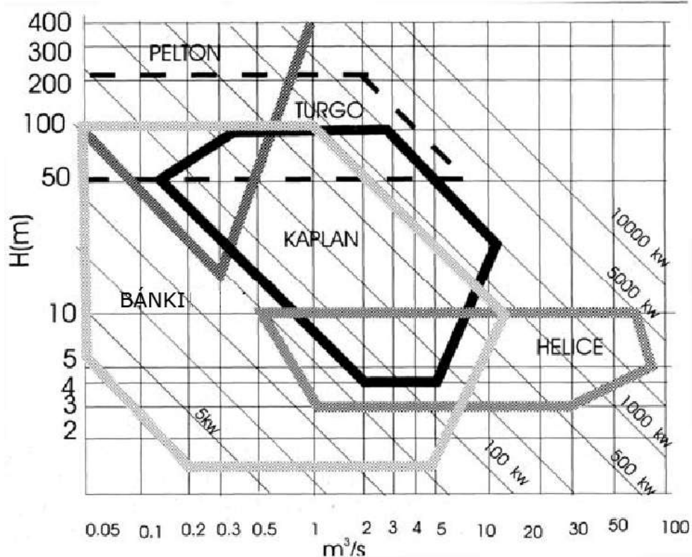
4. számú ábra: A különböző turbinafajták működési tartományai
