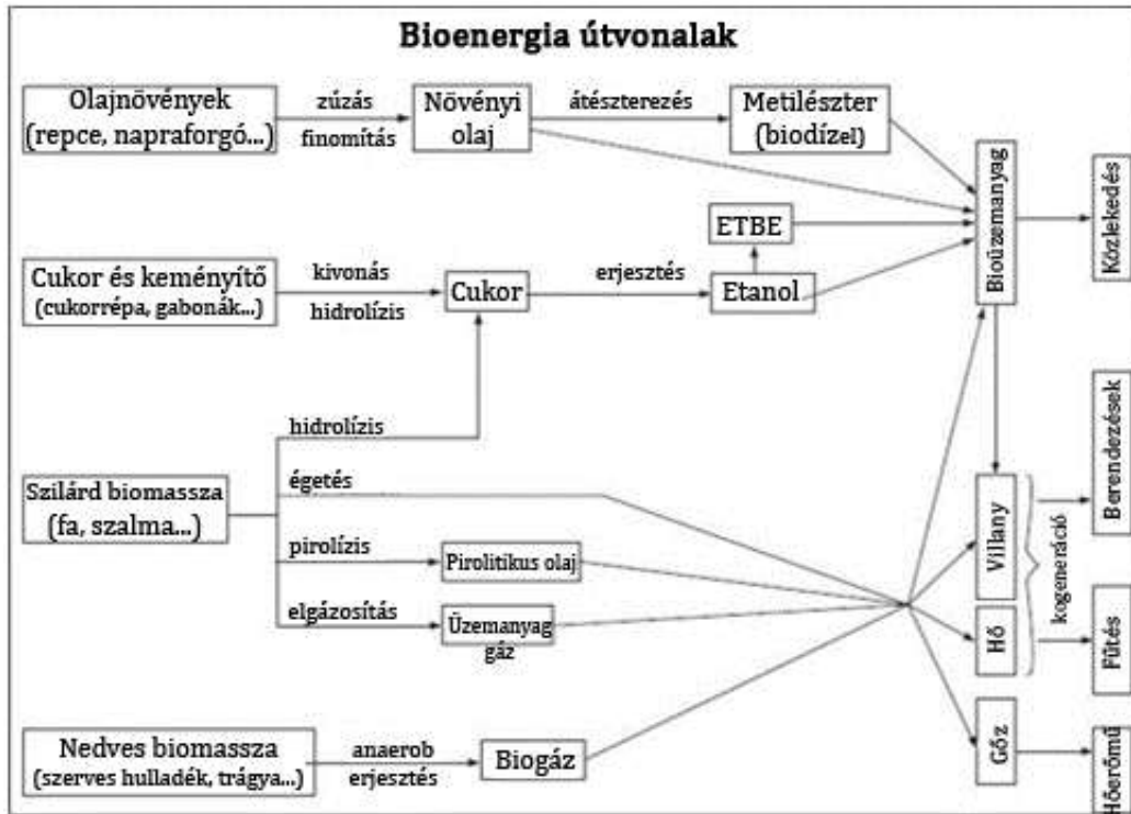
4. számú ábra – Biomassa technológiai rendszerek (EC, 2007).
