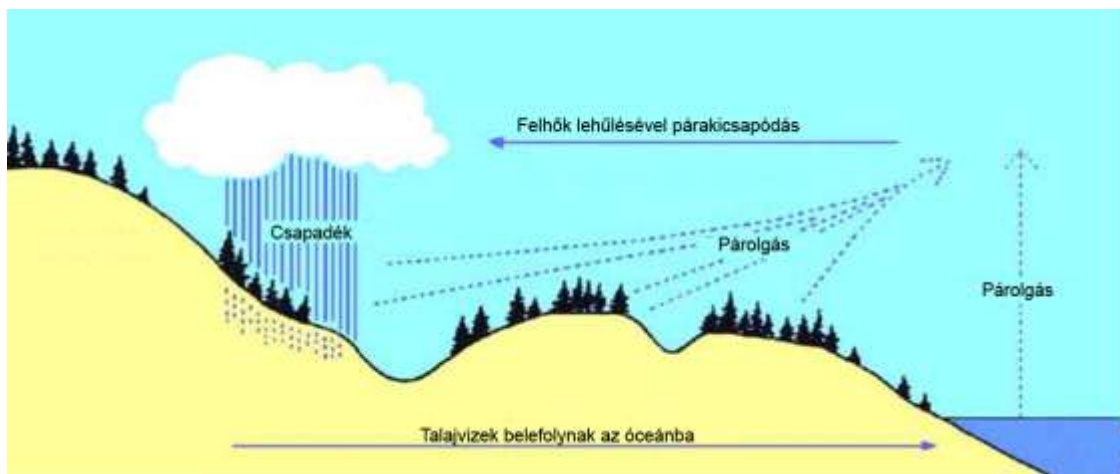
1. számú ábra: Vízkerforgás
