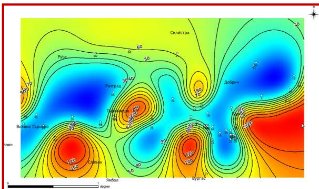
21. számú ábra - Az izotermákat 2500 méteres mélységben raszter interpolációval bemutató térkép
