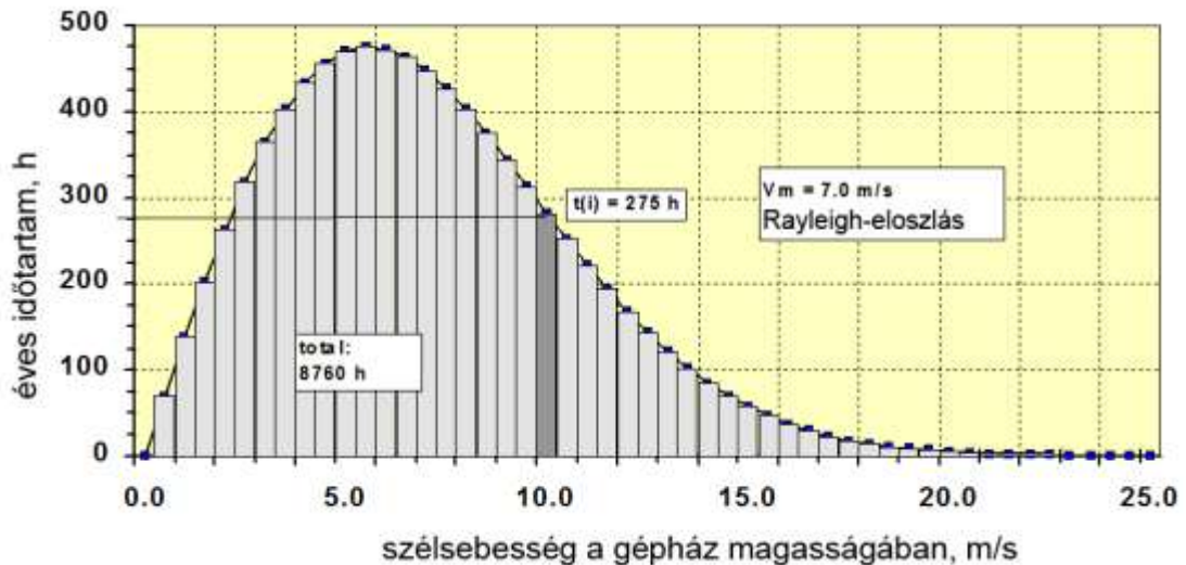
4.1. számú ábra: Példa mért szélesebbesség hisztogramjára ( v[i]=10.25 m/s; t[i]=275 h)
