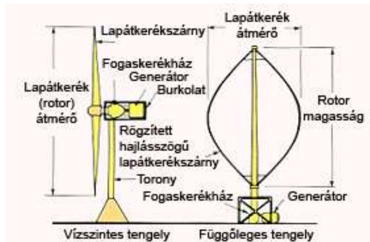
1.1. számú ábra: Szélturbina lehetséges kialakítási módjai
