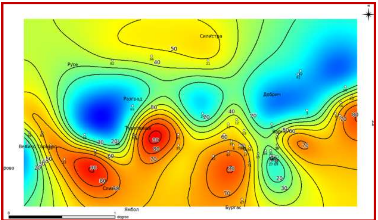
19. számú ábra - Az izotermákat 2000 méteres mélységben raszter interpolációval bemutató térkép
